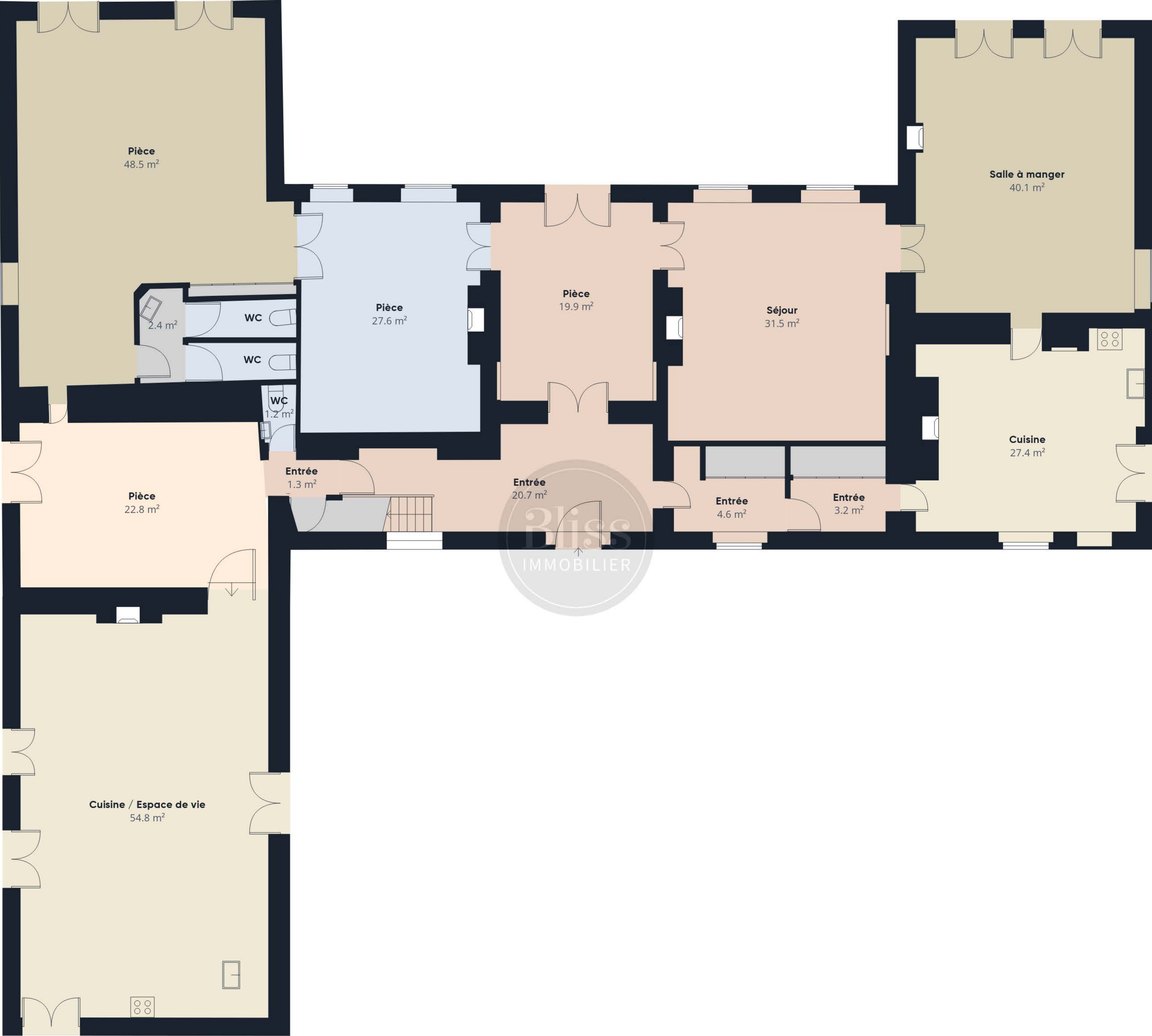
Niveau 0
